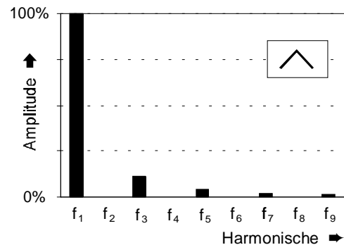
Abb. 4: Obertonspektrum einer Dreieck- welle
