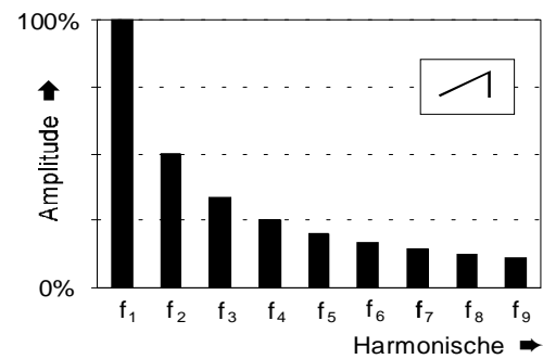
Abb. 1: Obertonspektrum einer Sägezahnwelle
